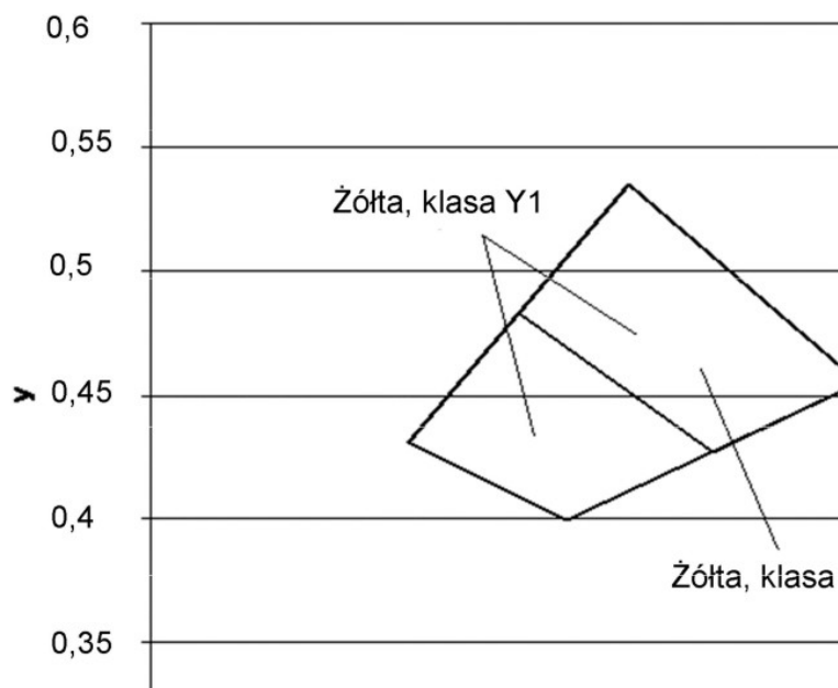
Rys.2. Współrzędne chromaticzności x,y dla barwy żółtej oznakowania
