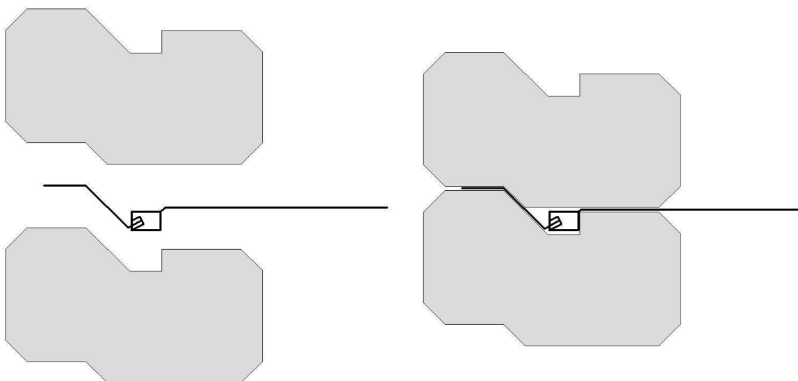
Rysunek 2. Prawidłowa długość swobodnego zębra po przycięciu georusztu
