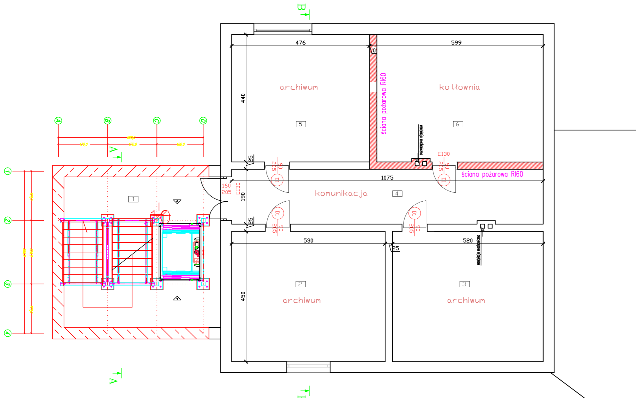
zestawienie pomieszczeń
