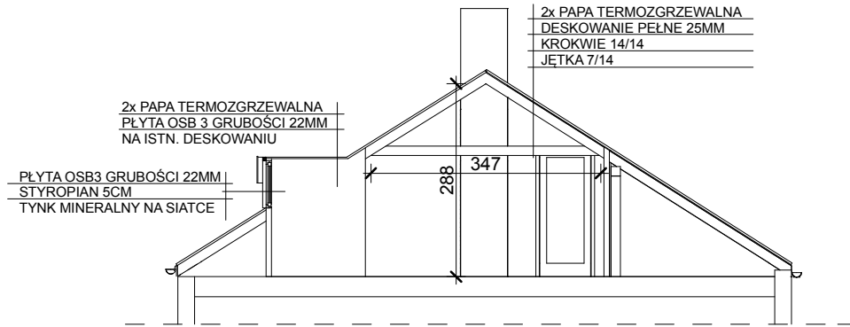
PRZEKRÓJ A-A 1:100
