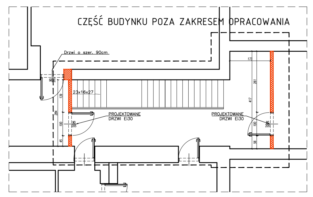
KORYTARZ NA POZIOMIE +1
