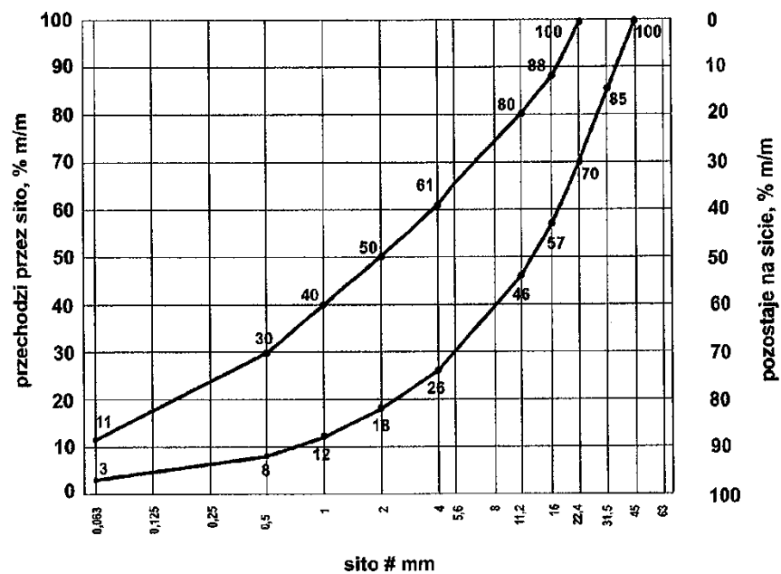
Rys. 1 Krzywe graniczne uziarnienia mieszanki mineralnej 0/31,5
