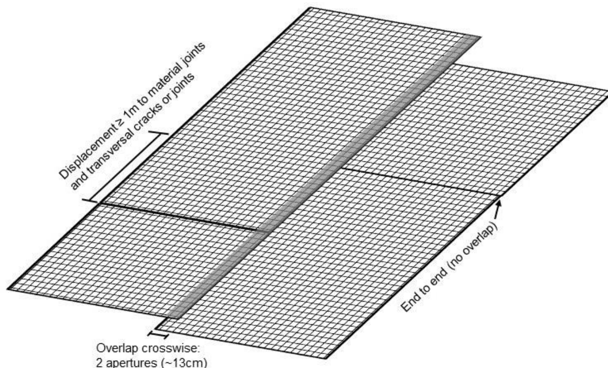
Rys. 1 Zasady instalacji kompozytu
