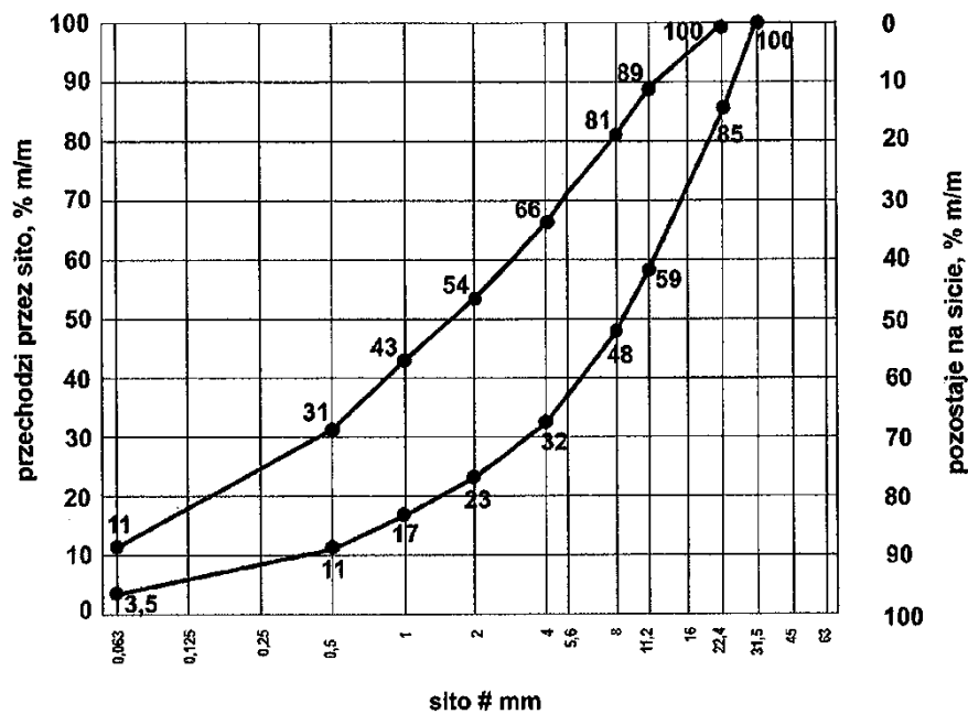
Rys. 2 Krzywe graniczne uziarnienia mieszanki mineralnej 0/22,4
