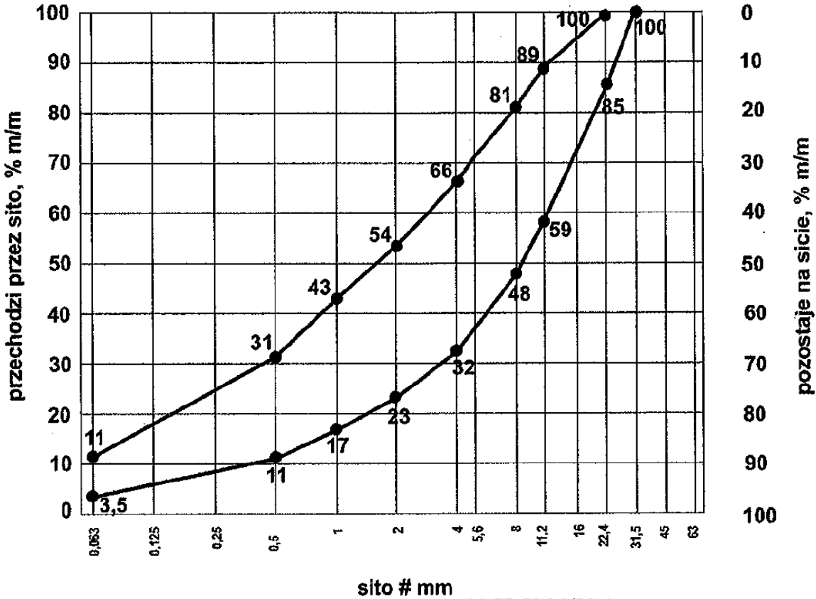
Rys. 1.2 Uziarnienie mieszanki CBGM 0/22,4
