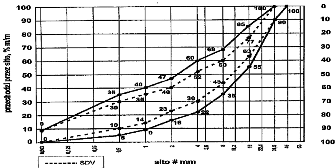
Rysunek 2. Uziarnienie mieszanki niezwiązanej 0/31,5 do podbudowy zasadniczej
