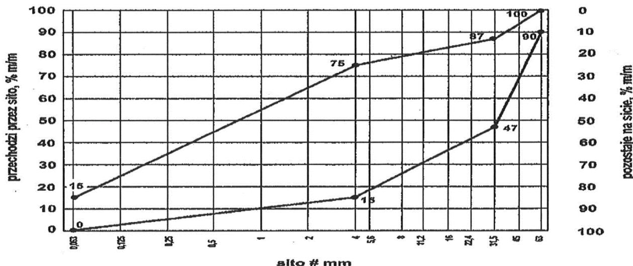
Rysunek 1. Uziarnienie mieszanki niezwiązanej 0/63 do warstwy mrozoochronnej
