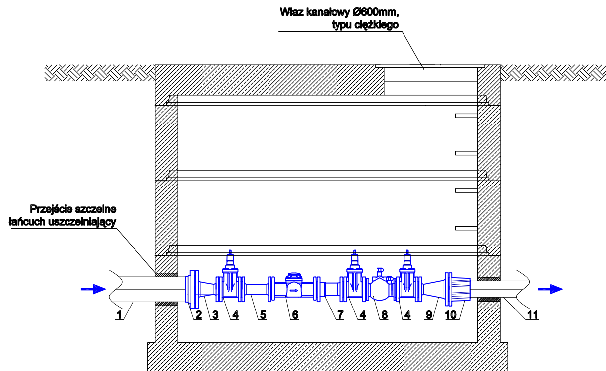
Rzekrój A-A studni wodomierzowej d=2000mm
