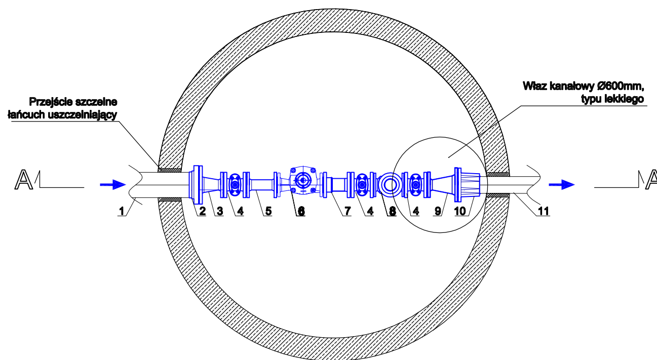
Rzut studni wodomierzowej d=2000mm
